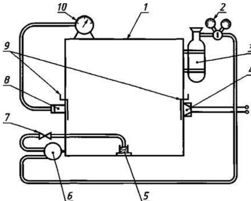
Рисунок 4 - Установка типа ОВИП
