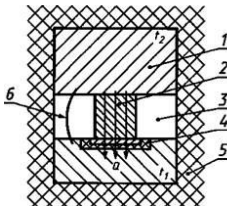
Рисунок 3 - Тепловая схема измерителя теплопроводности
