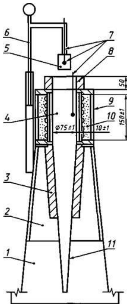
1 - подставка; 2 - вытяжка; 3 - теплоизоляционный слой защитного экрана и ста билизатора; 4 - трубчатая печь; 5 - держатель образца; 6 - устройство для опускания образца; 7 - термоэлектрические преобразователи; 8 - защитный экран; 9 - защитный кожух; 10 - теплоизоляционный материал; 11 - стабилизатор воздушного потока
